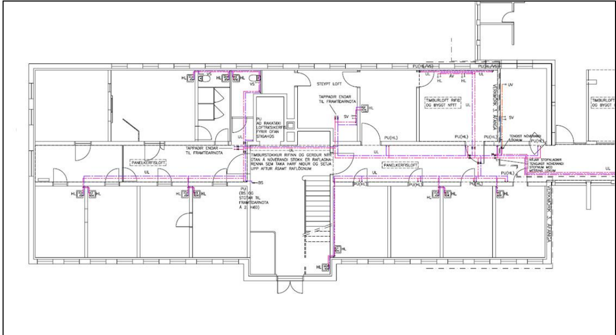
Grunnmynd 1. hæðar A-álfu. Teikning Tækniþjónustu SÁ.ehf.
