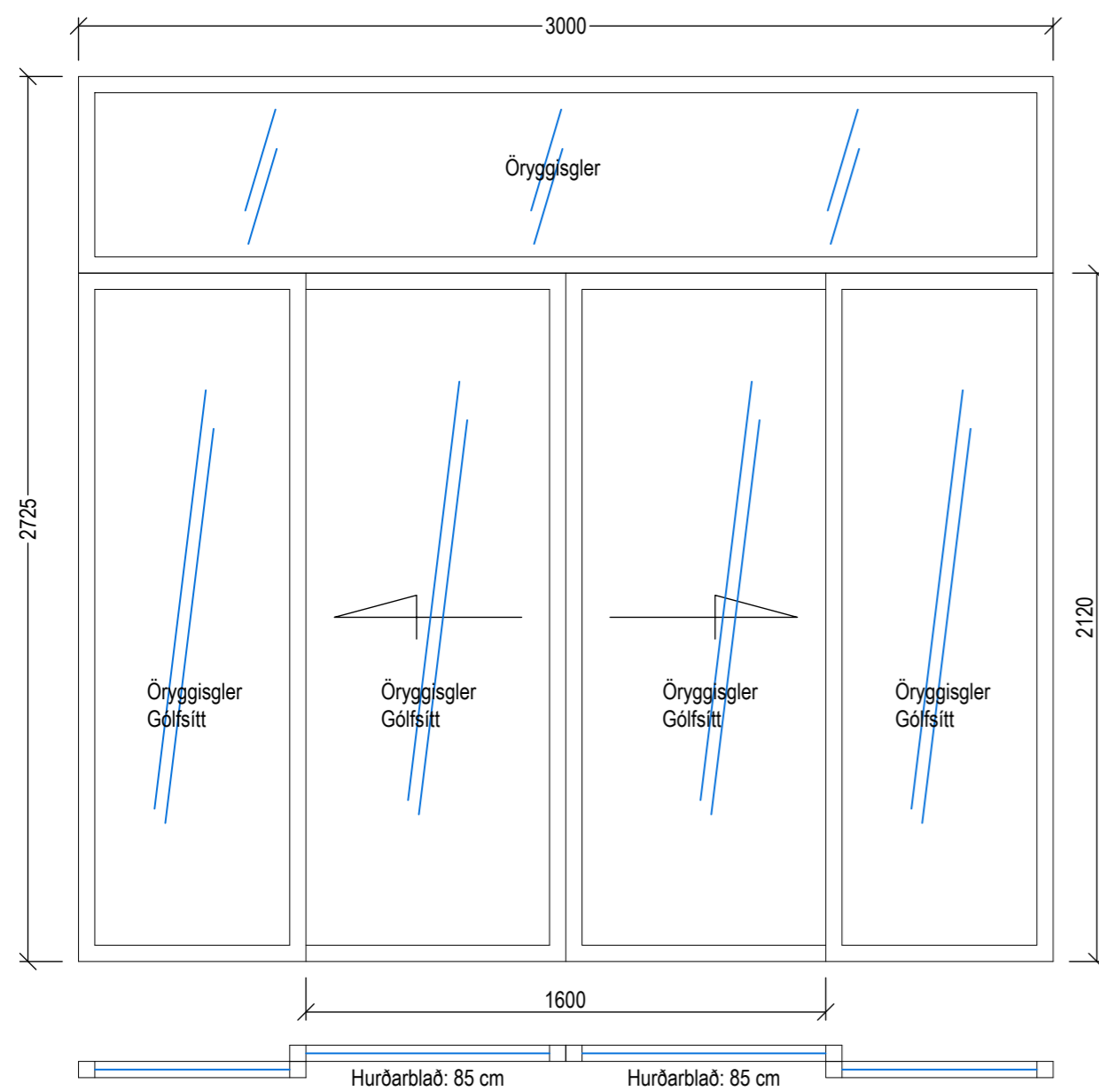
ÚH-01 - 1 Stk Mkv = 1:20
