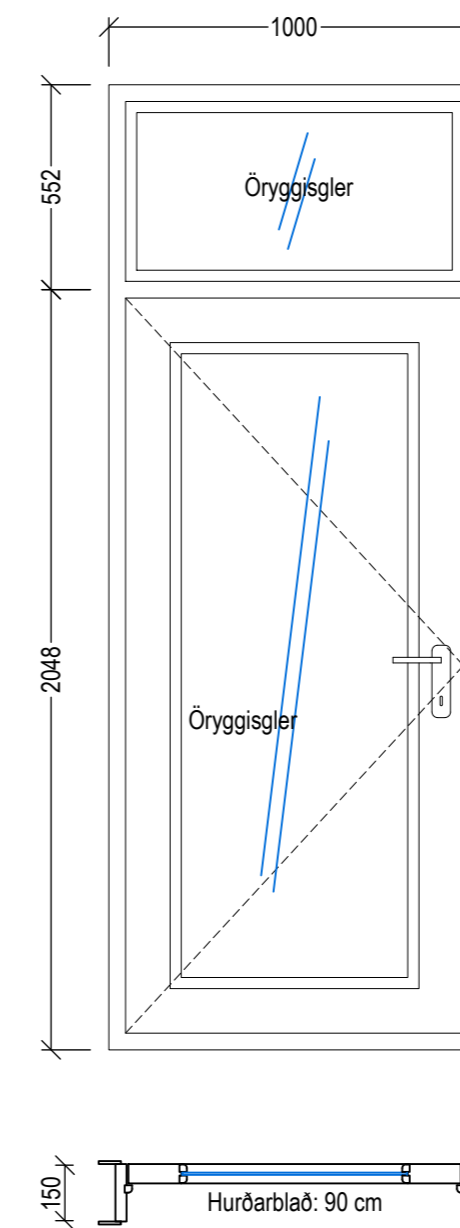
ÚH-03 - 1 Stk Mkv = 1:20
