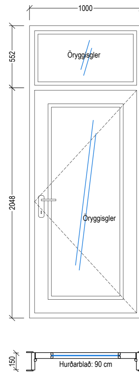
ÚH-02 - 2 Stk Mkv = 1:20
