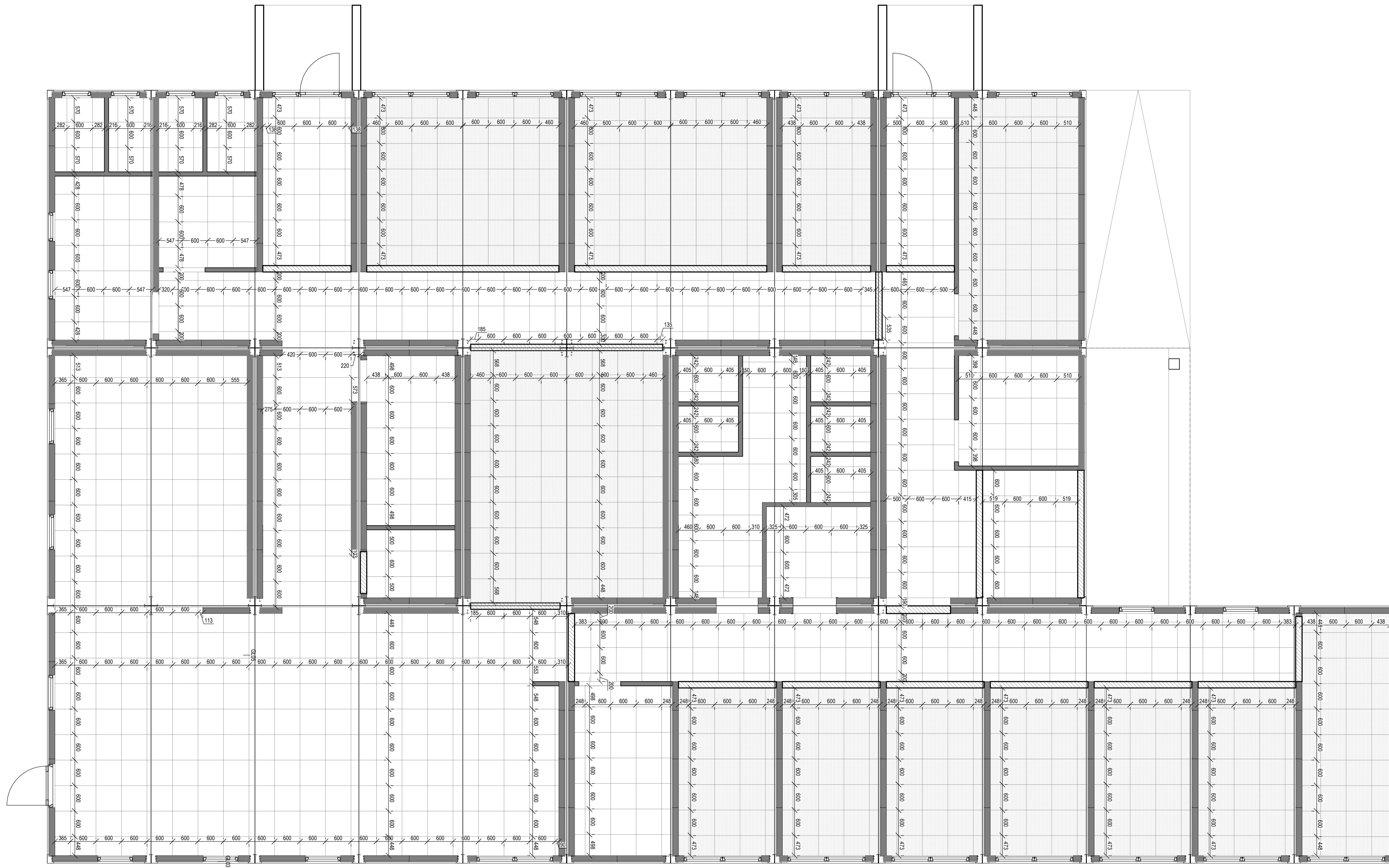
Grunnmynd - niðrhengt loft M= 1:50
